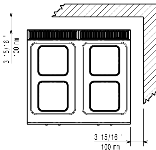
Boven aanzicht
